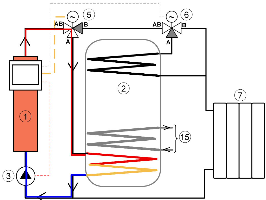
2. Накопление тепла: нагреватель греет теплоаккумулятор.
