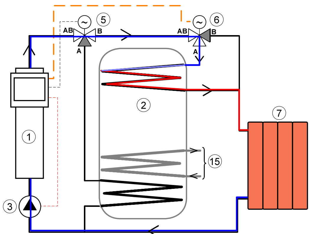
3. Экономия: аккумулятор греет радиаторы. Нагреватель выключен.
