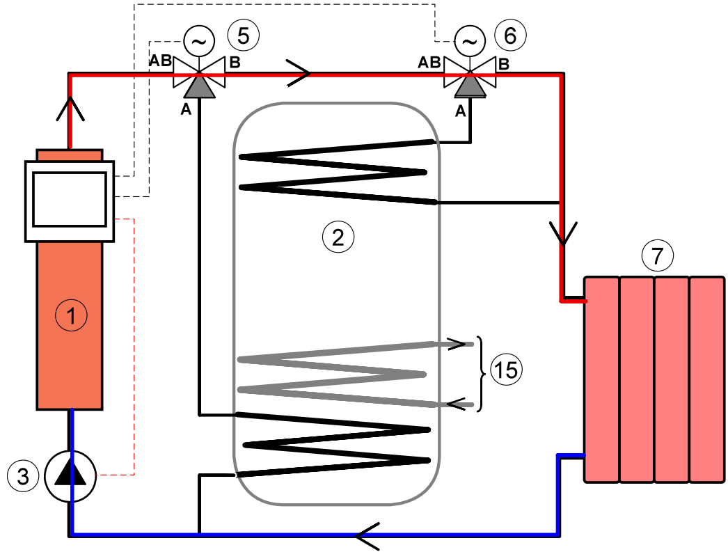
1. Отопление: нагреватель греет радиаторы.
